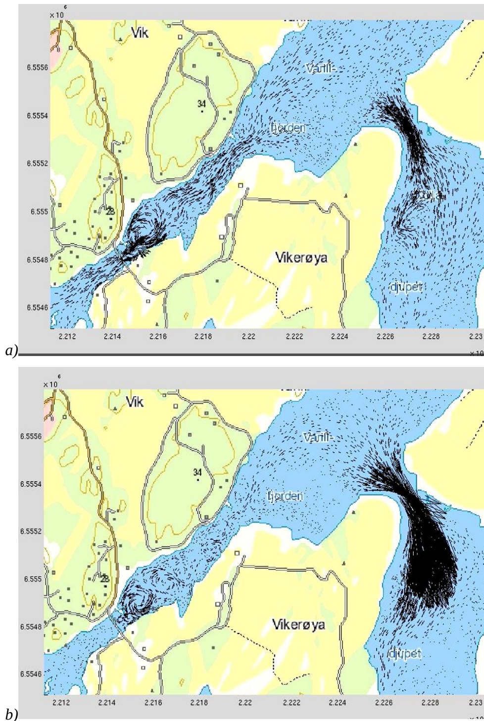
Figur 11: Illustrasjoner av stillbilder fra simuleringer med FVCOM ved a) stigende sjø med åpen tidevannsport og b) fallende sjø med lukket tidevannsport. Pilene viser strømretning. Lengden på pilene viser relativ styrke på strømmen.
