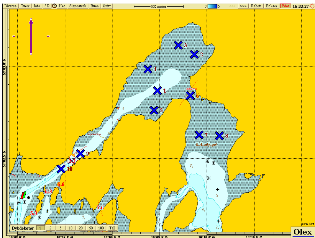
Figur 8: Oversikt over de 10 stasjonene (blå kryss og med tall) hvor det ble sluppet ut partikler i FISC-simuleringene (kartverktøy: www.olex.no ).
