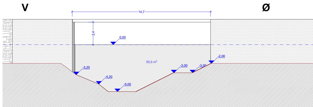
Figur 24: Skisse av tverrsnittet over Vikørøybrua, med diverse dyp, bredder og areal. Merk at dette kun er en foreløpig og grovt forenklet skisse (kilde: IT-Tek).
