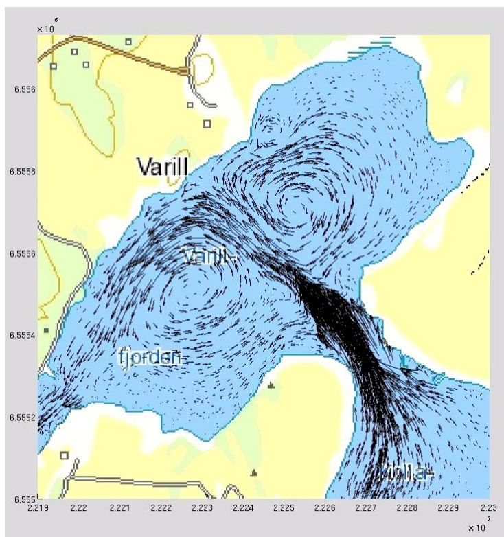
Figur 22: Stillbilde fra Varildfjorden ved simulering med den hydrodynamiske modellen FVCOM. Det er her kjørt med tidevannsport ved Vikørøybrua som lukkes ved innstrømmende tidevann. Det blir da satt opp en kraftig strømjett i Klåstadrenna, som vil kunne danne virvler innover i den nordlige delen. Virvlene vil være positivt for omrøring og utskifting av vannmasser.
